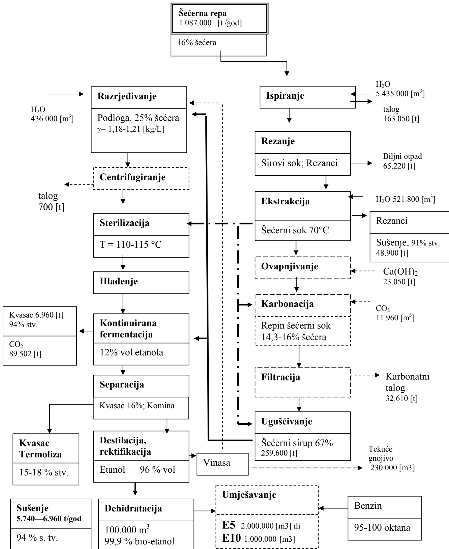
Slika 7.3 Shema proizvodnje 100.000 [m 3 /god] bio-etanola iz šećerne repe za E5 i E10 gorivo
